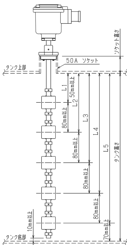
接点参考図
