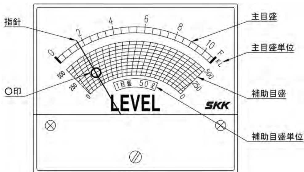
ファインインジケーターの例（タンク容量：10kL）
