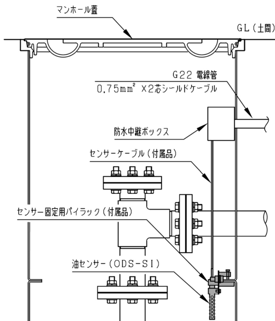
地下タンクサンプ内設置図
