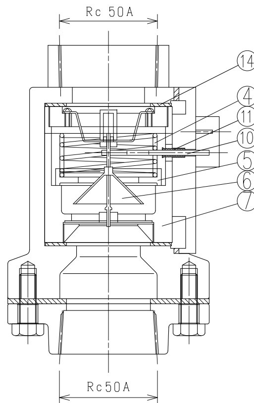
A-A断面図
