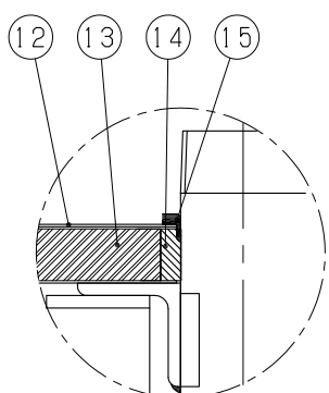
A部詳細
