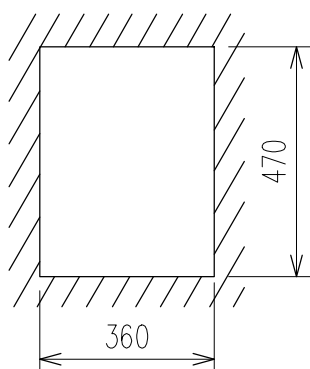
パネルカット寸法
