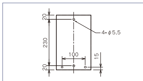
屋內壁掛け型
