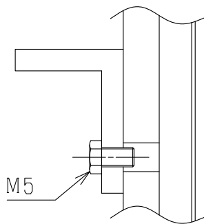
A部詳細
