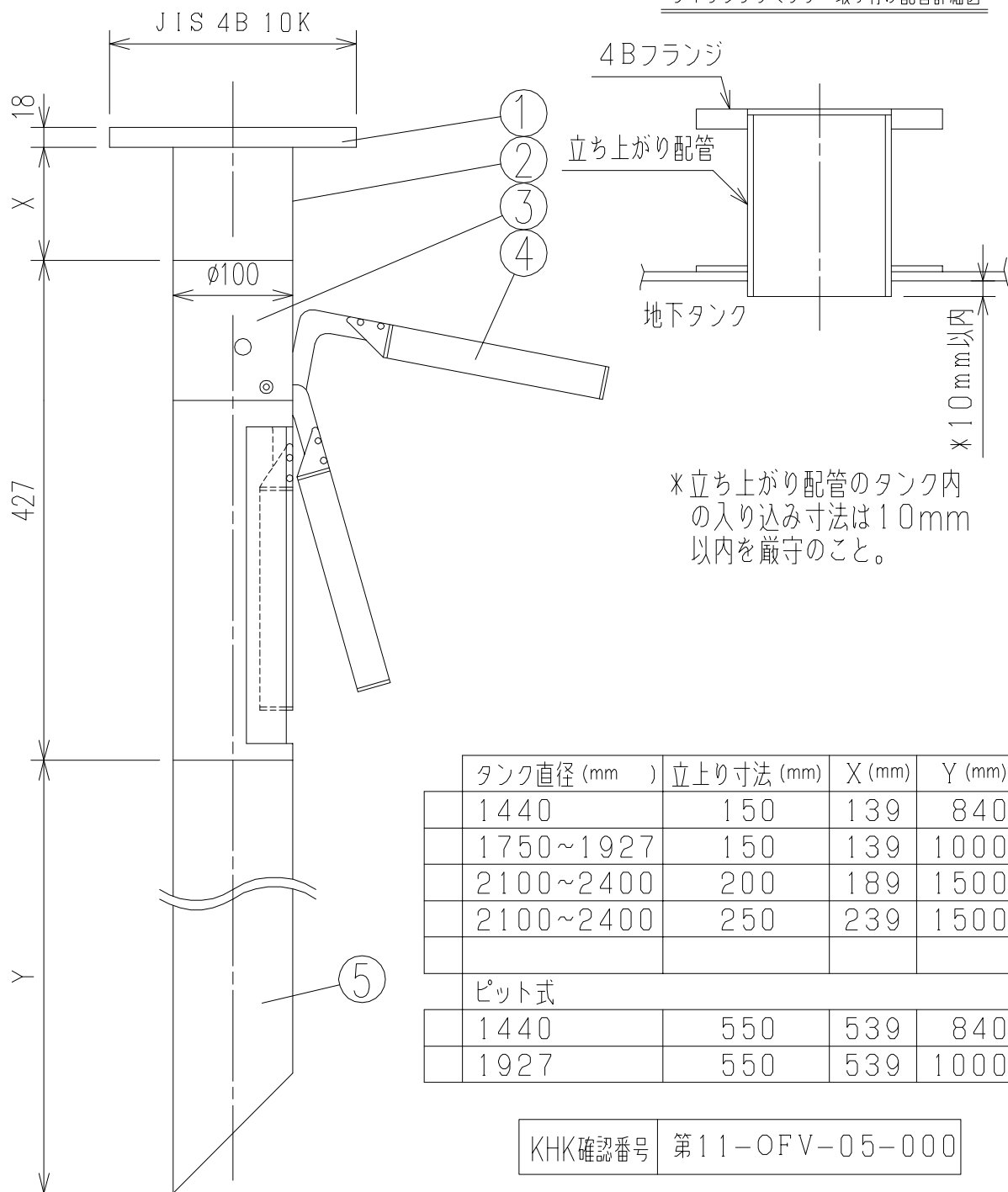
フィリングリミッター取り付け配管詳細図
