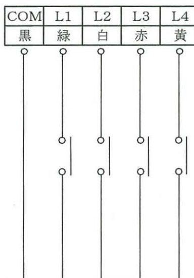
端子台配列および内部回路
