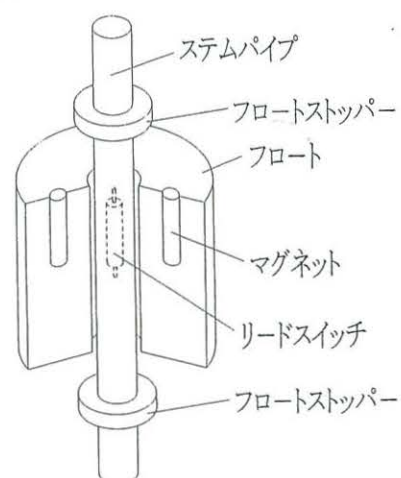
構造図
