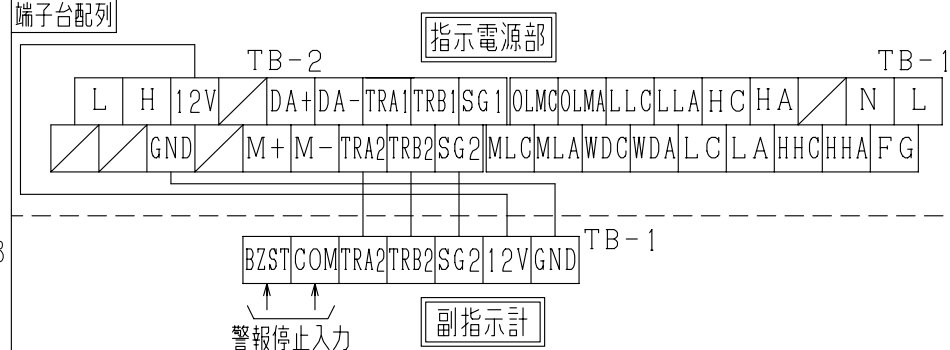
端子台配列
