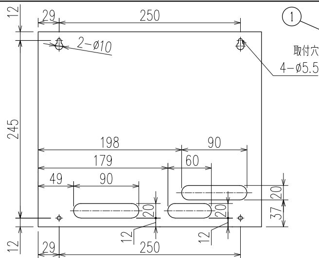
背面取付穴および入線孔図
