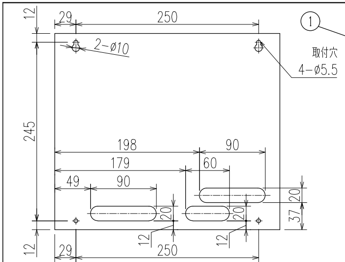
仕 様 背面取付穴および入線孔図
