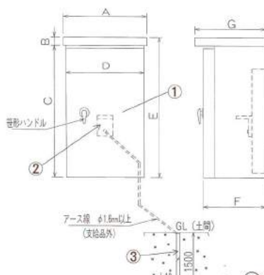
型式 RAB-160
