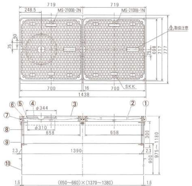
MS-2100-WN型 (安全荷重50kN)
