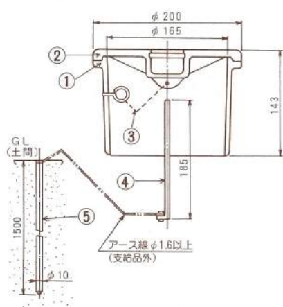
型式 RAB-160
